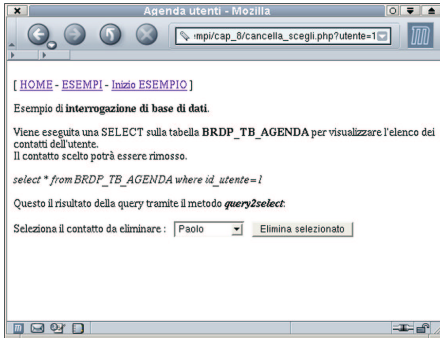
Figura 7.8. Tramite questa pagina è possibile scegliere il contatto da rimuovere.
