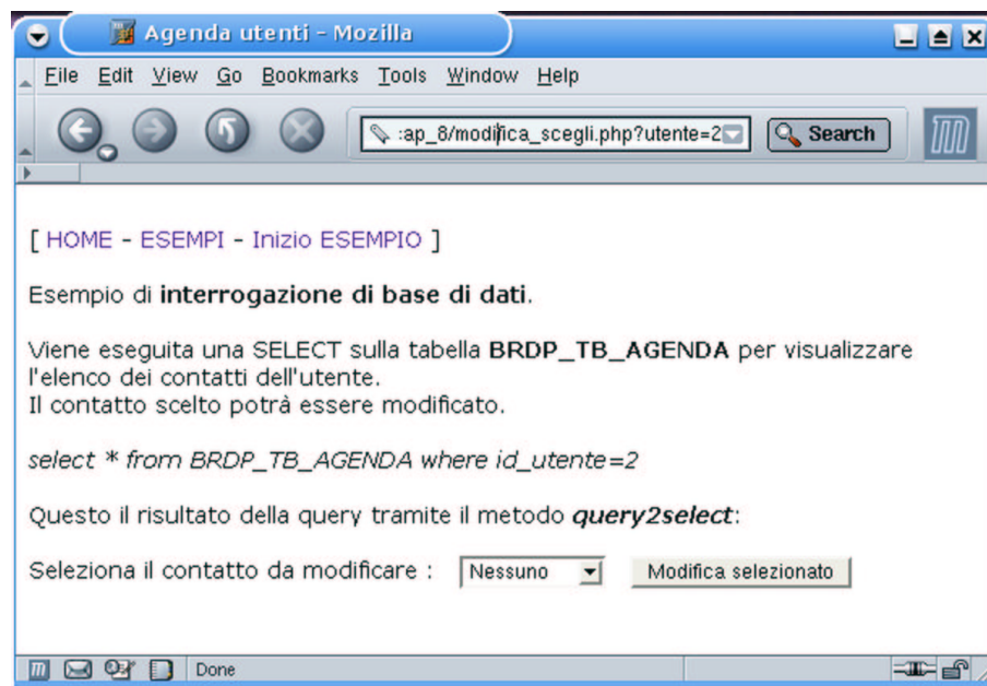
Figura 7.10. Del tutto simile a cancella_scegli.php ; a cambiare è la pagina di destinazione modifica_modifica.php .
