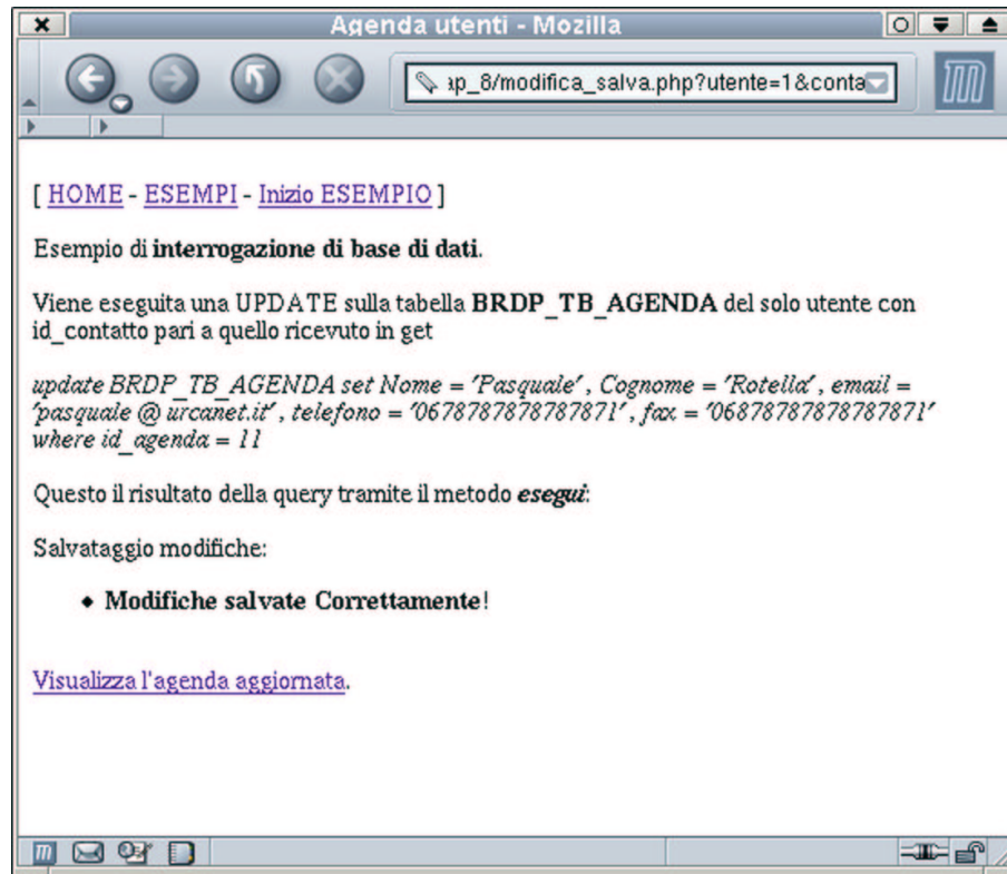
Figura 7.12. Viene visualizzata la query e mostrato l'esito della sua esecuzione.
