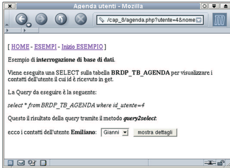
Figura 7.3. Il metodo query2select esegue la query e restituisce direttamente valori in una SELECT HTML.
